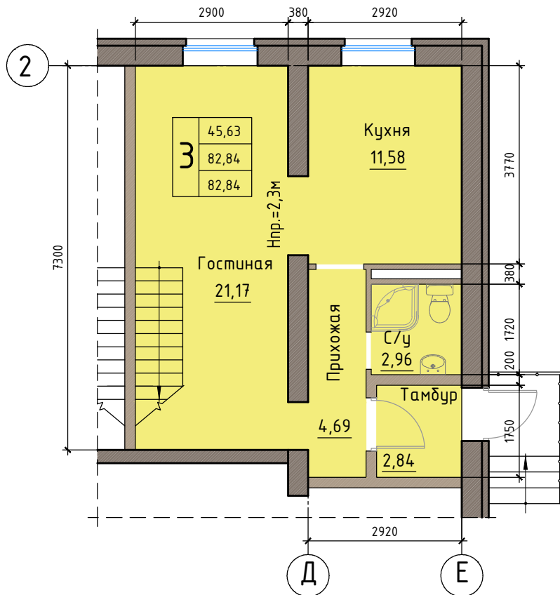
Блокировочная схема дома №2
