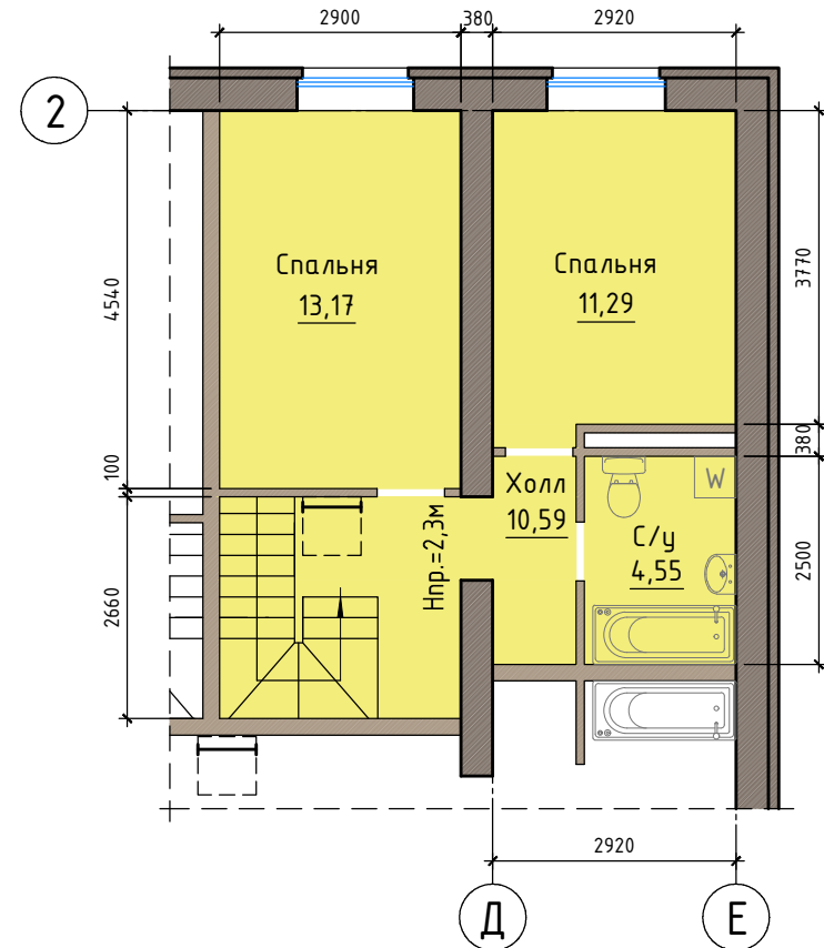
План 2 этажа
