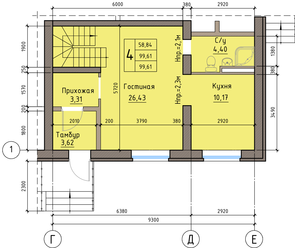
Блокировочная схема дома №2
