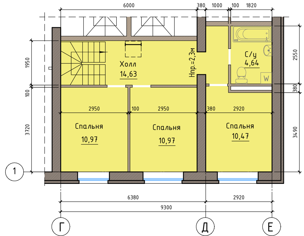
План 2 этажа
