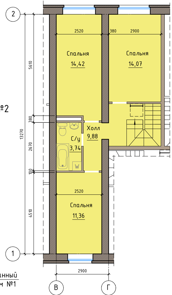
План 2 этажа
