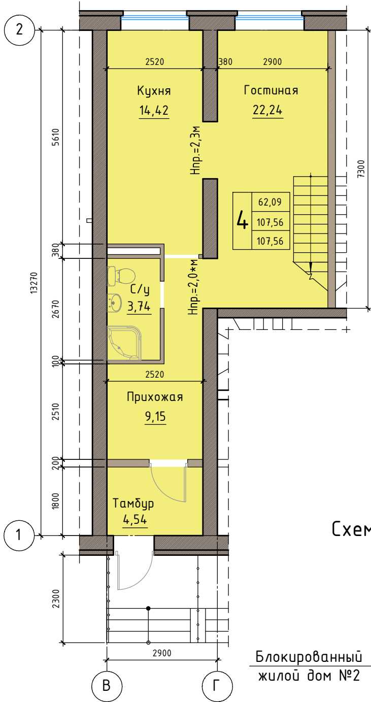
План 1 этажа
