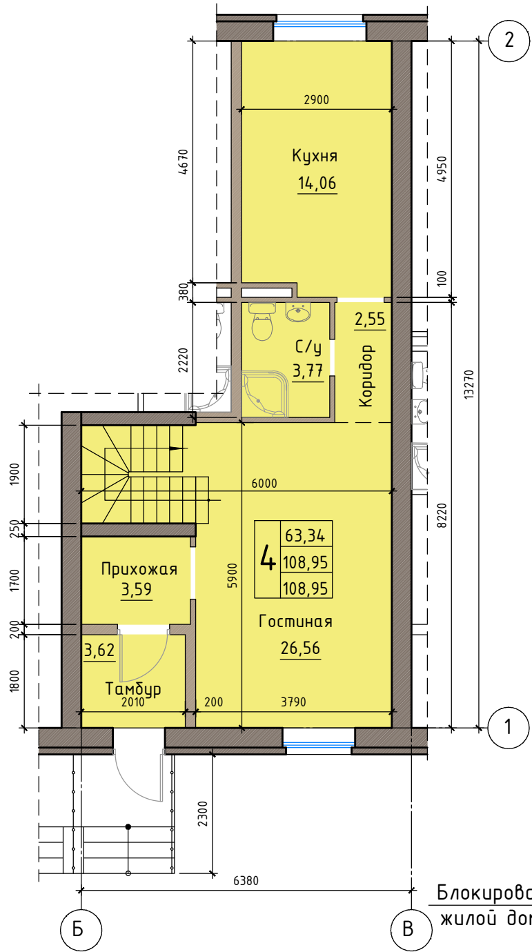
План 1 этажа
