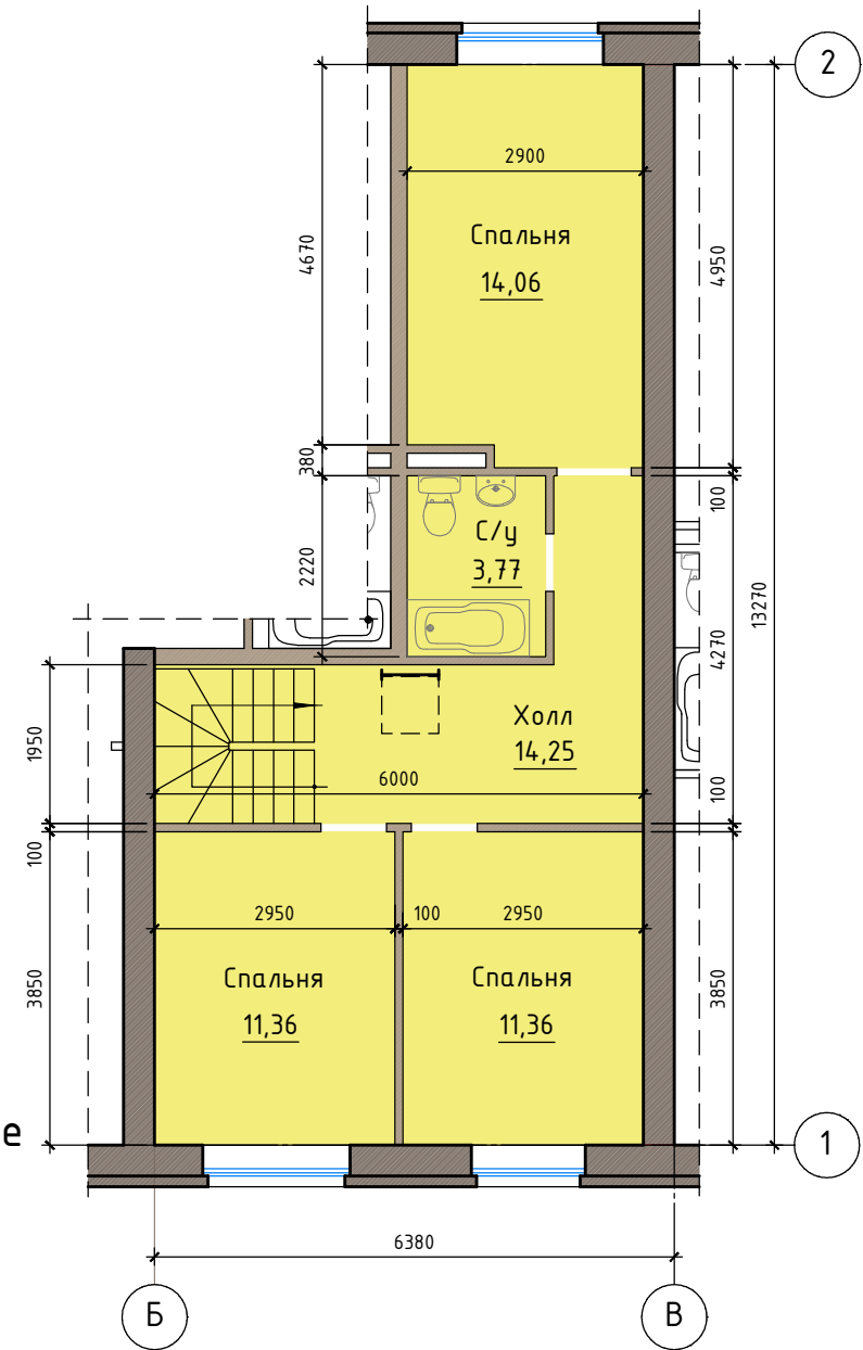
План 2 этажа
